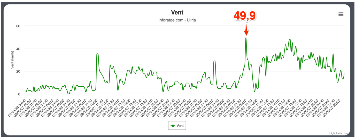
Ráfagas de viento registradas en LLÍRIA los días 02 y 03/09/23 (en km/h) https://inforatge.com/meteo-lliria
