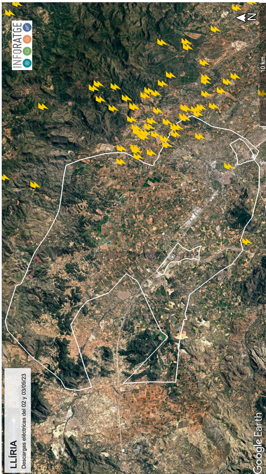
Geolocalización de las descargas eléctricas «nube-tierra» registradas en el término municipal de LLÍRIA los días 02 y 03/09/23 Fuente descargas eléctricas: AEMET Agencia Estatal de Meteorología // Cartografía: © Instituto Geográfico Nacional de España
